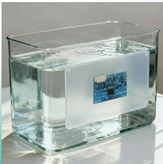
Implementazione contenitore removibile Sensore applicato su parete non a contatto con il contenitore (possibile gap di aria)
